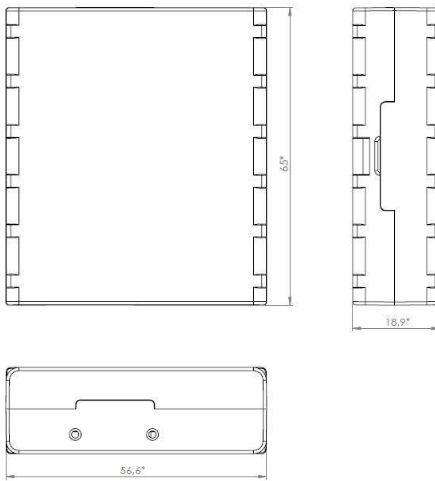
Рис. 1. Внешний вид и размеры FMA110 (точность \pm 2 мм).
