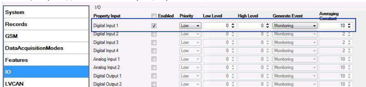
Рис. 41. Конфигурирование I/O параметров.
