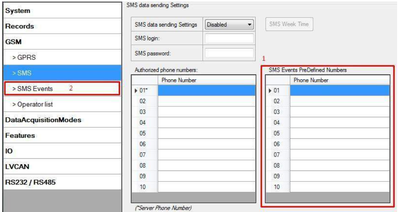
Рис. 33. Список заданных телефонных номеров (SMS Events PreDefined Numbers).
